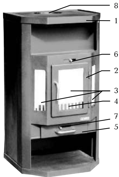
Рис. 1г. Печь-камин "ВОЛГА" (АОТ-9-01)
