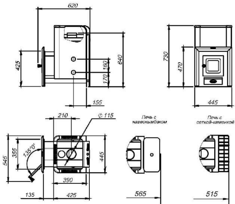
Рисунок - 5а. Габаритные и установочные размеры печи-каменки.
