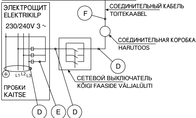
Подключение в 3-фазной сети, 230V 3~ Kerise 3-faasilised elektri hendused, 230V 3~
