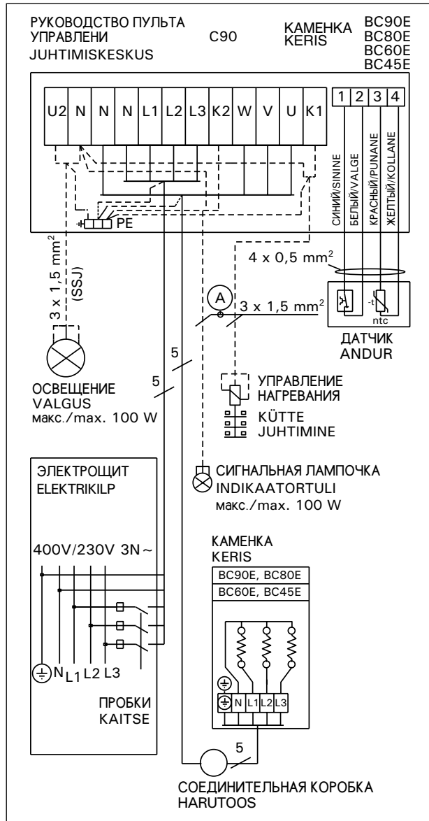
Рисунок 11 с. Электромонтаж пульта управления C90 и каменки ВСЕ (подключение в 3-фазной сети) Joonis 11с. Juhtimiskeskuse C90 ja BCE-kerise 3-faasilised elektri hendused
