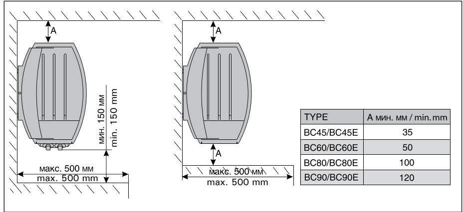
Рисунок 6. Установка каменки в нишу Joonis 6. Kerise paigaldus seinas vendisse
