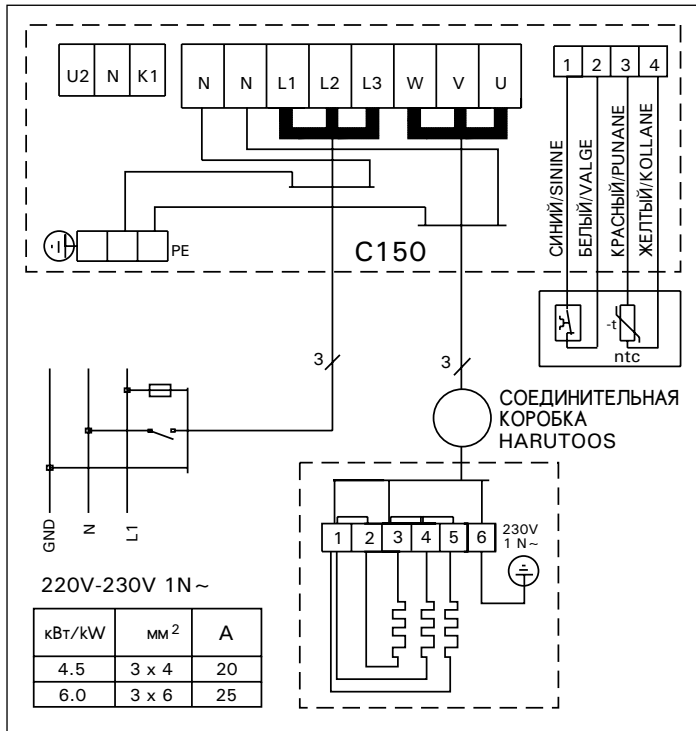
Рисунок 11 а. Электромонтаж каменок BC45E и BC60E для российского рынка (подключение в 1-фазной сети) Joonis 11a. Keriste BC45E ja BC60E 1-faasilised elektri hendused
