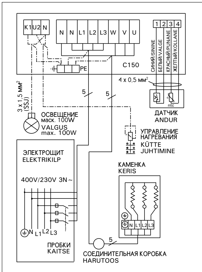
Рисунок 11 б. Электромонтаж пульта управления C150 и каменки ВСЕ (подключение в 3-фазной сети) Joonis 11b. Juhtimiskeskuse C150 ja BCE-kerise 3-faasilised elektri hendused
